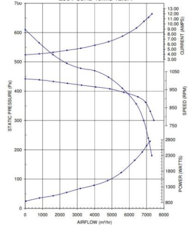
TORIN SIFAN AFZUIGMOTOR 7000 M3/H DDC381-286-1400W-6P-1SP 230V 50Hz 40Mfd 12.0A
